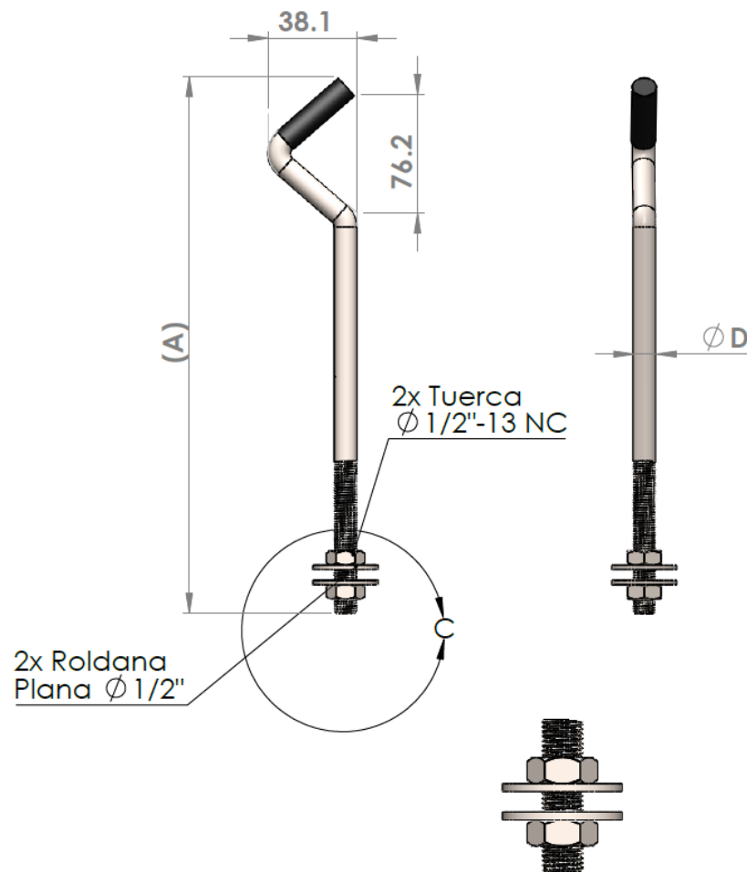
DETALLE C ESCALA 2 : 3.8
